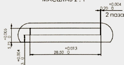
ЭЛЕМЕНТ С 2 места МАСШТАБ 2 : 1
