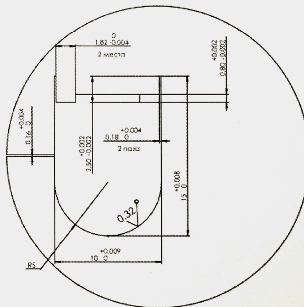
ЭЛЕМЕНТ А МАСШТАБ 5 : 1
