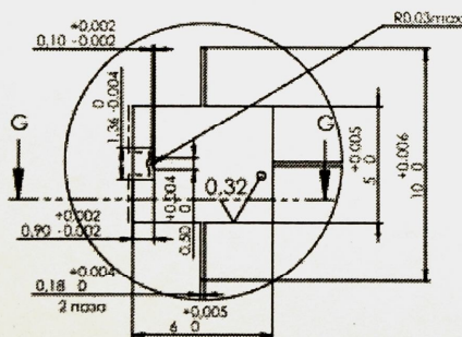
СЕЧЕНИЕ G-G МАСШТАБ 5 : 1
